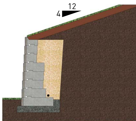
Oppervlak bovenaan keerwand met helling van 18° [4/12] - geen overlast
