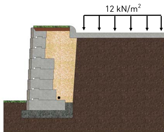
Oppervlak bovenaan keerwand zonder helling - 12 kN/m² overlast
